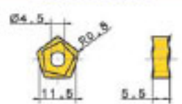
PNCU0805GNTR
